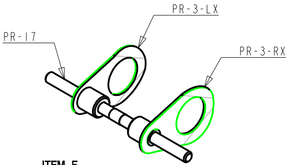
ITEM 5 PR-3-XX LEFT & RIGHT EDGE GUIDE ASSY
